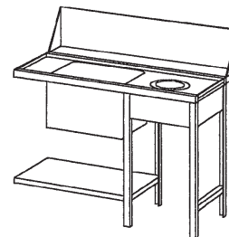
Vorbräuerung rechts mit Abfallschacht, mit Spritzschutz, 100 mm hoch Spülbecken links B 1200 x T 720 x H 850 mm Gewicht: 21 kg GTIN (EAN) 4015613371863 | Art.-Nr. 109773 | Euro 1.149,-
