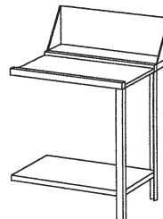
Zu- oder Ablauftisch rechts mit Spritzschutz, 100 mm hoch B 700 x T 720 x H 850 mm Gewicht: 15 kg GTIN (EAN) 4015613371887 | Art.-Nr. 109776 | Euro 489,-
