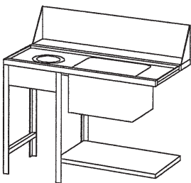
Vorbräuerung links mit Abfallschacht, mit Spritzschutz, 100 mm hoch Spülbecken rechts B 1200 x T 720 x H 850 mm Gewicht: 21 kg GTIN (EAN) 4015613371856 | Art.-Nr. 109772 | Euro 1.149,-
