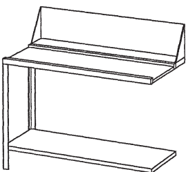
Zu- oder Ablauftisch links mit Spritzschutz, 100 mm hoch B 1200 x T 720 x H 850 mm Gewicht: 17 kg GTIN (EAN) 4015613371894 | Art.-Nr. 109777 | Euro 689,-
