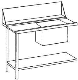
Vorbräuerung links mit Spritzschutz, 100 mm hoch Spülbecken rechts B 1200 x T 720 x H 850 mm Gewicht: 19 kg GTIN (EAN) 4015613370675 | Art.-Nr. 109770 | Euro 1.068,-
